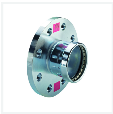
Prestabo XL karimás átmeneti idom SC-Contur-ral (biztonsági kontúr) modellszám 1159XL cikkszám 598 235
